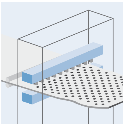
Breitpresse
