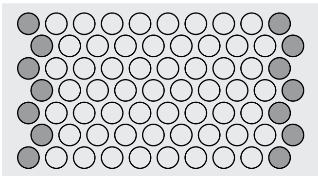
Normal versetzte Lochreihen (vollständiges Lochbild)
