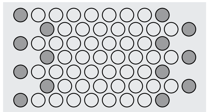
Doppelt versetzte Lochreihen (unvollständiges Lochbild)
